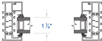
SECTION A-A: JAMBS
